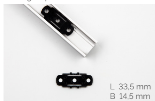
Montageclips
